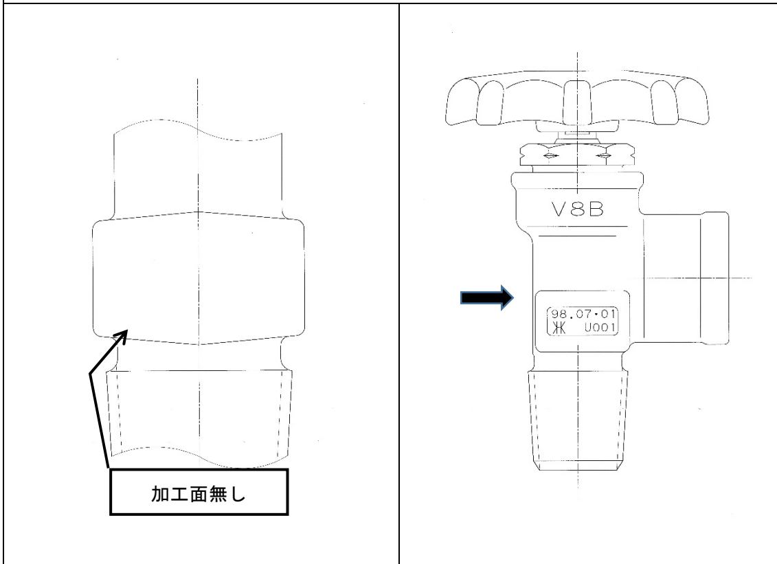
新鍛造ボディ（V-8B 専用鍛造品）
