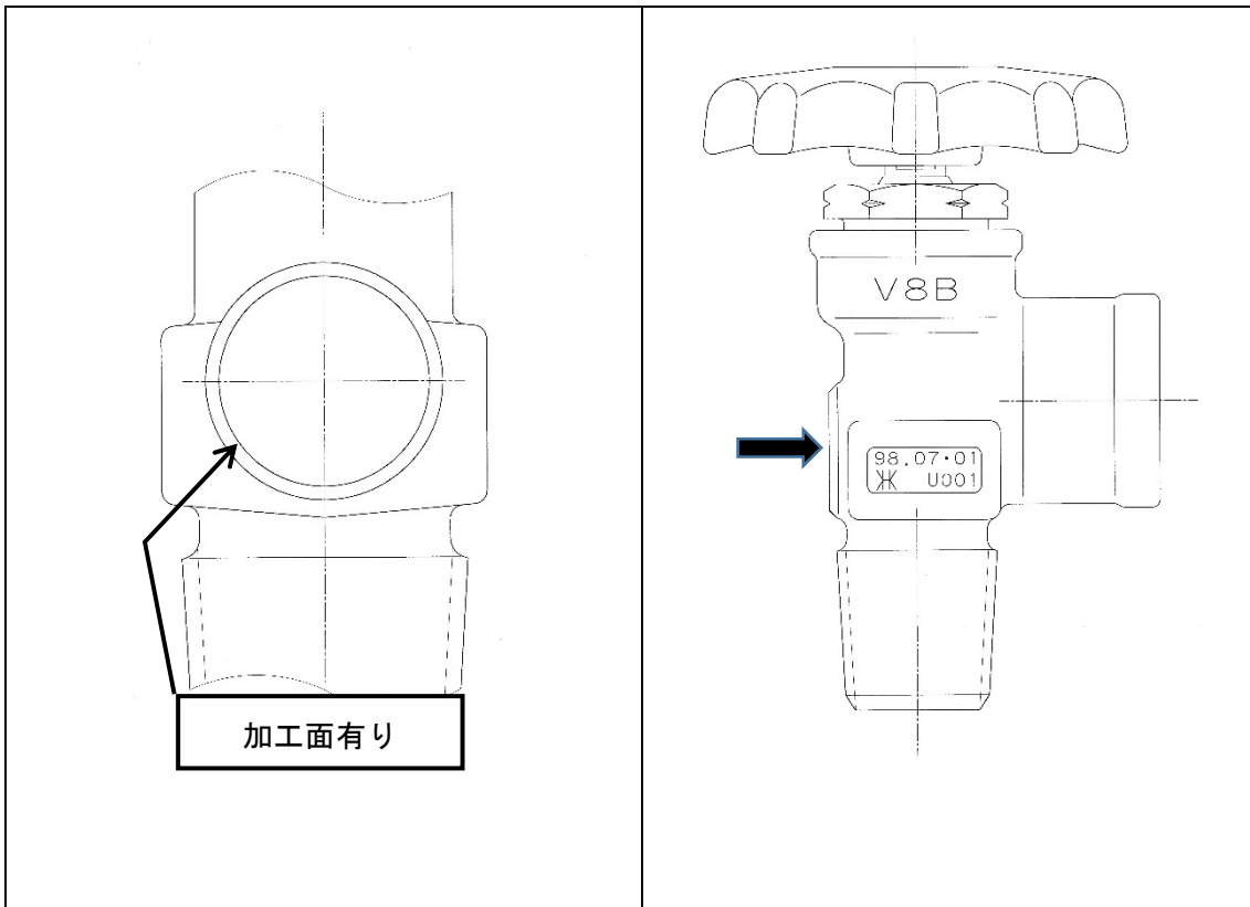
旧鍛造ボディ（V-8 鍛造ボディ加工共用品）
